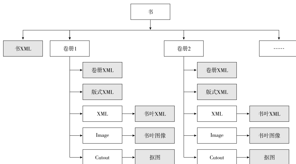
图 1 汉文古籍版式描述数据存储目录结构示意图
